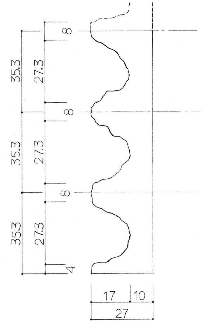
A-A 断面詳細図
